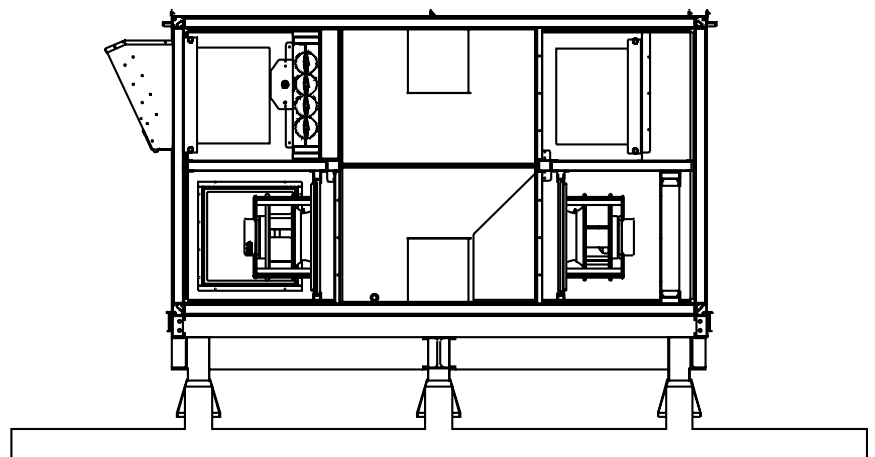
C-C ( 1 : 15 )
